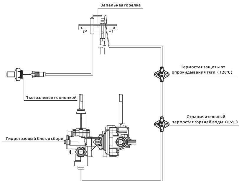
Рис.2. Схема электрическая
