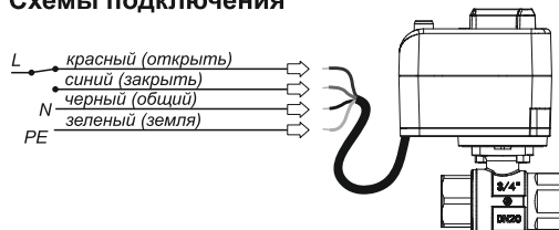
Электрическая схема подключения крана с электроприводом серии Neptun Profi Click 230B (рис. 3)
