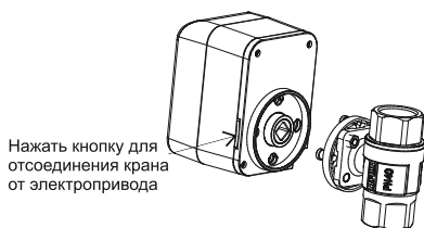
Способ фиксации арматуры (рис. 2)
