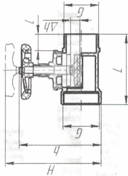
Рисунок 1 – Внешний вид клапанов угловых моделей КЛЛ, КЛЧ, КПК и КЛЛМ, КЛЧМ, КПКМ
