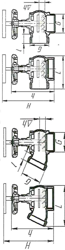
Рисунок 1 – Внешний вид клапанов угловых моделей КПЛ, КПЧ, КПК и КПЛМ, КПЧМ, КПКМ Исполнение 1: КПЛМ, КПЧМ, КПКМ, КПЧМ, КПКМ, КПКМ, КПКМ Исполнение 2: КПЛ, КПЧ, КПК
