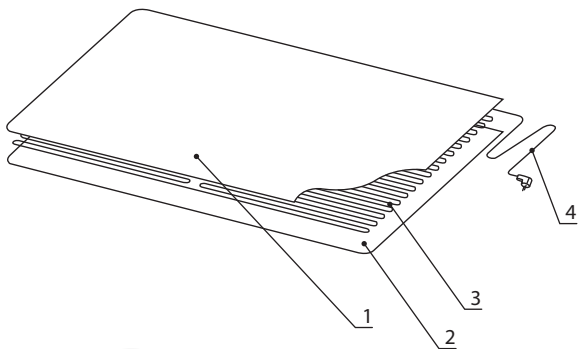
Рис. 1. Конструкция нагревателя
