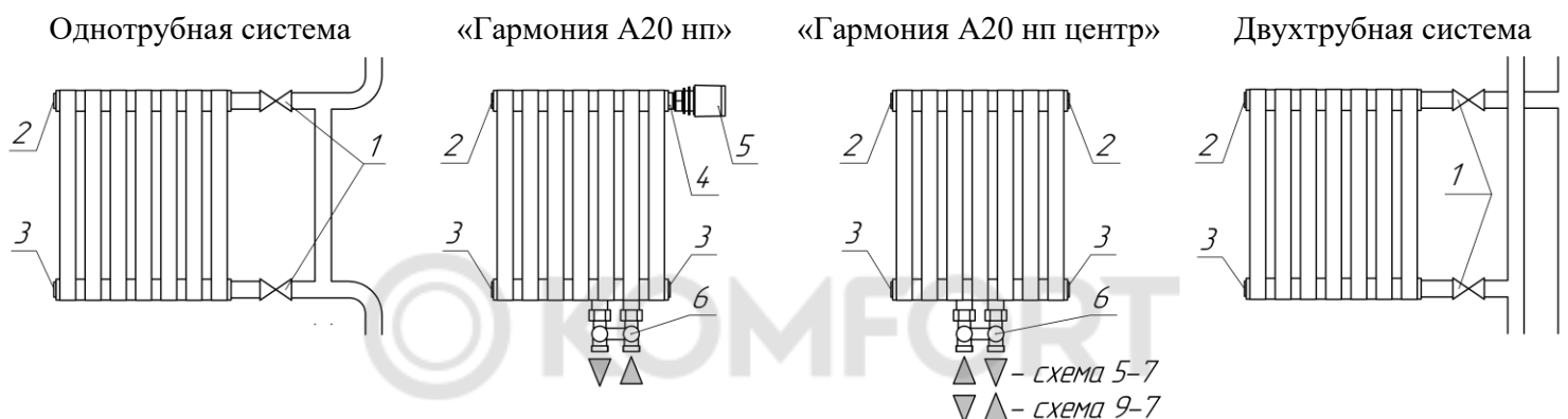
Рис. 2 1. Вентиль. 2. Кран Маевского-воздухоотводчик. 3. Пробка глухая (точка слива). 4. Встроенный термоклапан. 5. Термостатический элемент. 6. Запорно-присоединительный клапан нижнего подключения.
