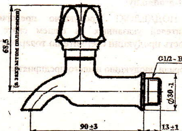
Рисунок 1. Кран КрН15
