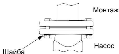
Рис. 3 Положение шайб для овальных отверстий под болты
