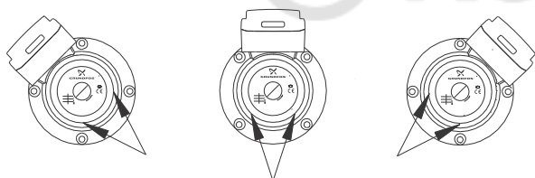
Рис. 5 Расположение клеммной коробки у одинарных насосов
