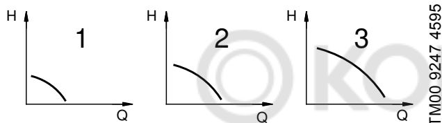
Рис. 10 Характеристика насоса на скорости 1, 2 и 3
