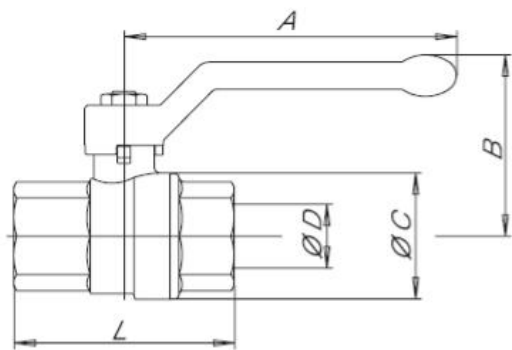
Рис. 1. Габаритные и присоединительные размеры
