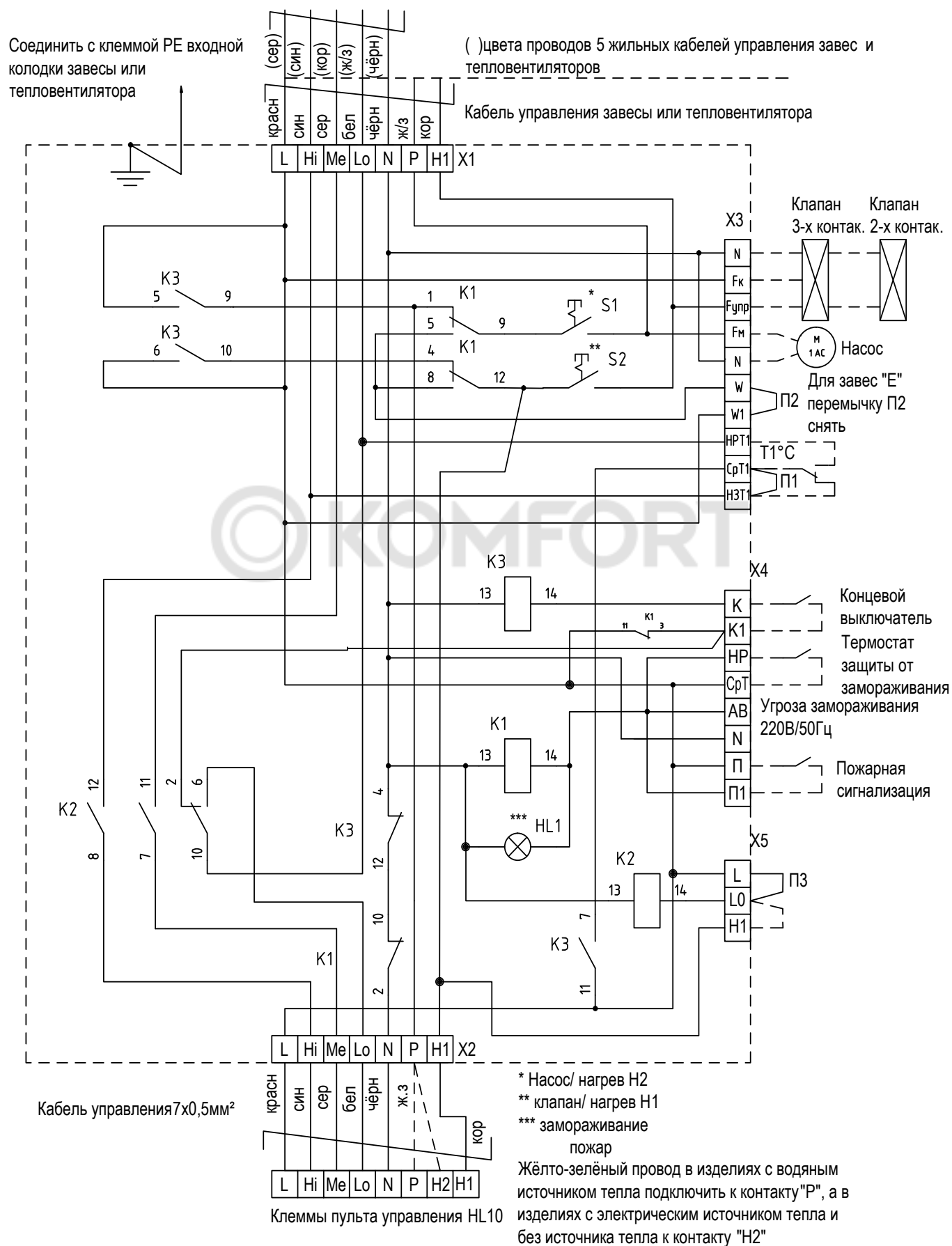
Рисунок 1. Электрическая схема БЛОК-WA (ver.E)
