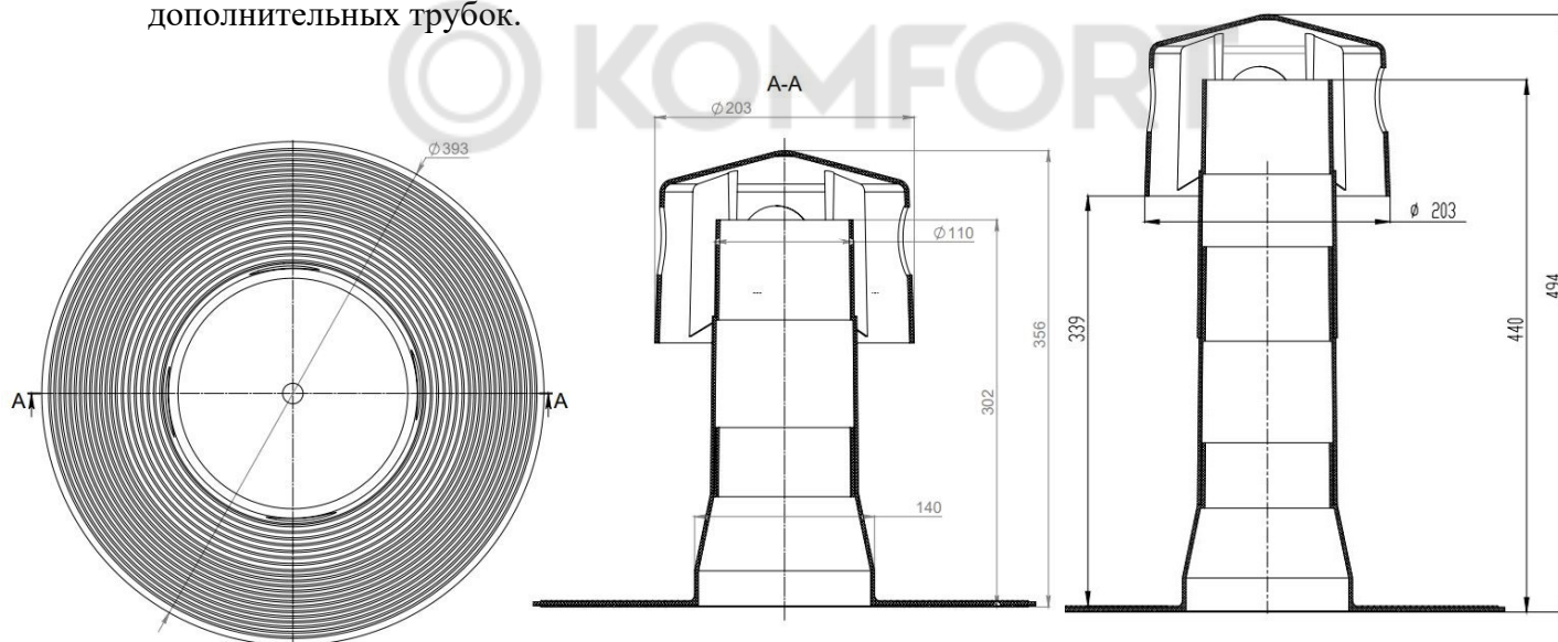
Рис. 1. Схема аэратора
