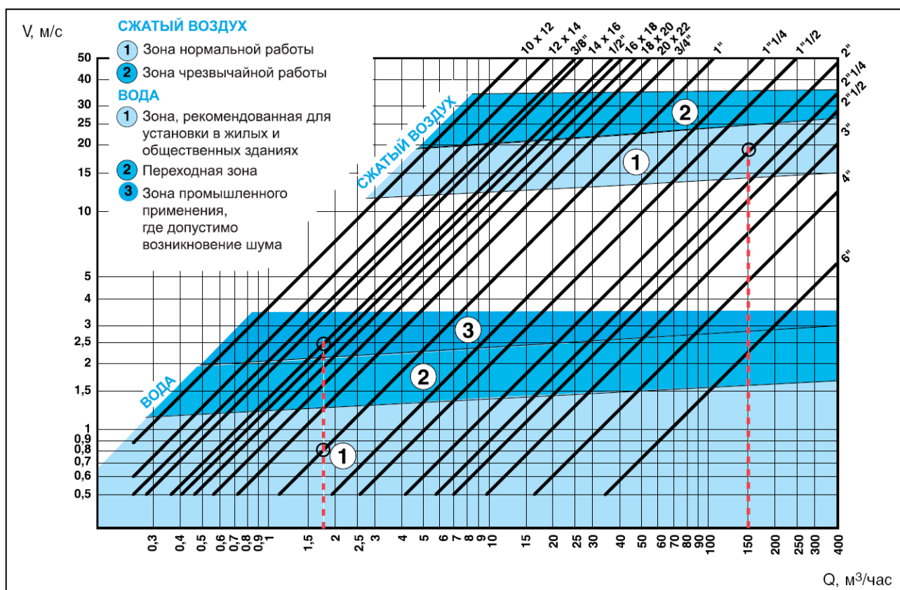
Рис. 2 Номограмма для подбора диаметра редукционного клапана.
