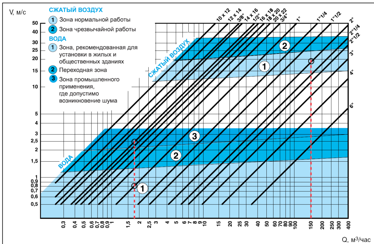
Рис. 2 Номограмма для подбора диаметра редуционного клапана.
