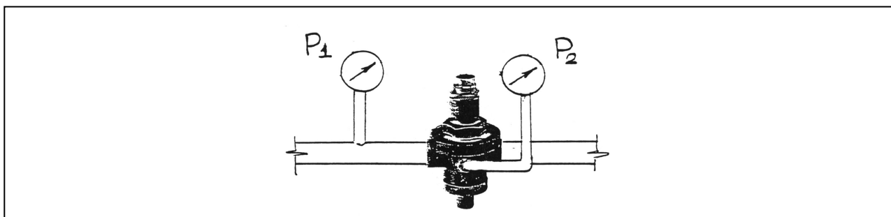
Рис. 4 Схема для настройки клапана.
