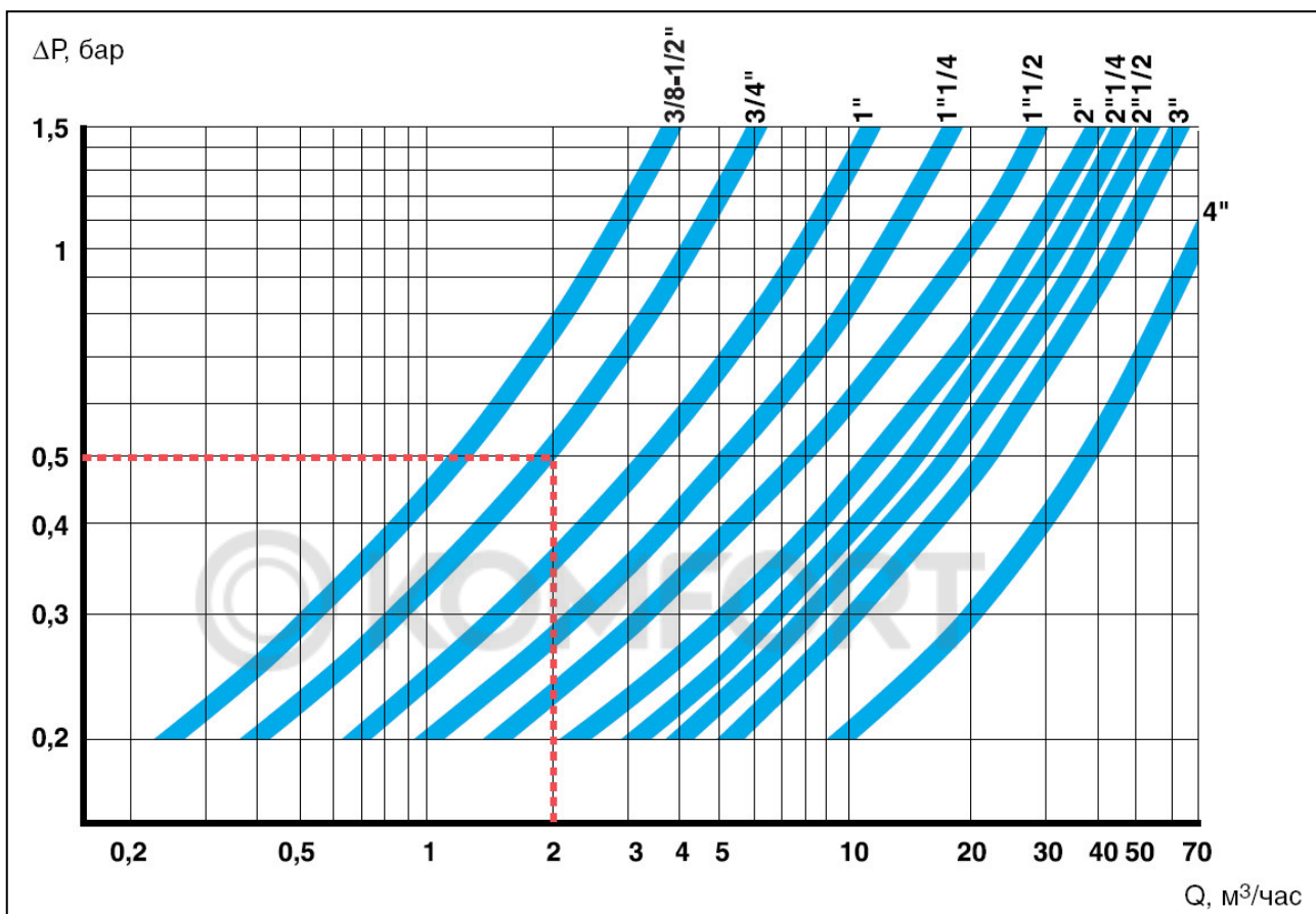
Рис. 3 Номограмма потерь давления.
