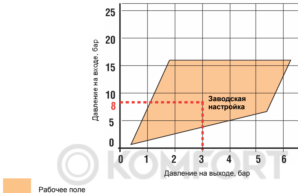
Рис. 1 Диапазон регулирования давления.
