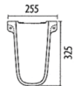
вид сверху
