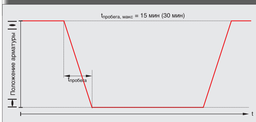
Типичная характеристика режима управления
