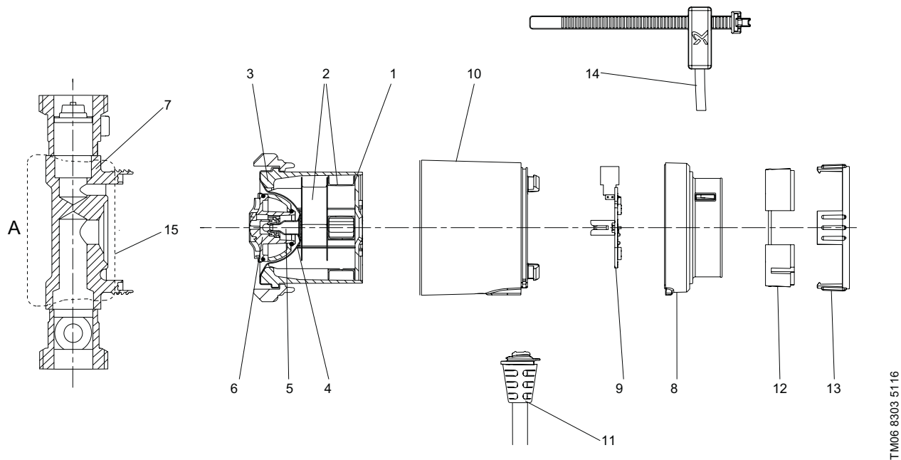
Рис. 16 Чертёж насоса COMFORT
