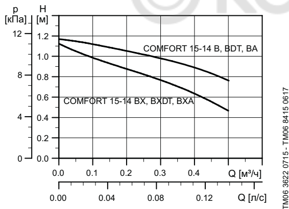
Рис. 2 Расходно-напорная характеристика насосов COMFORT
