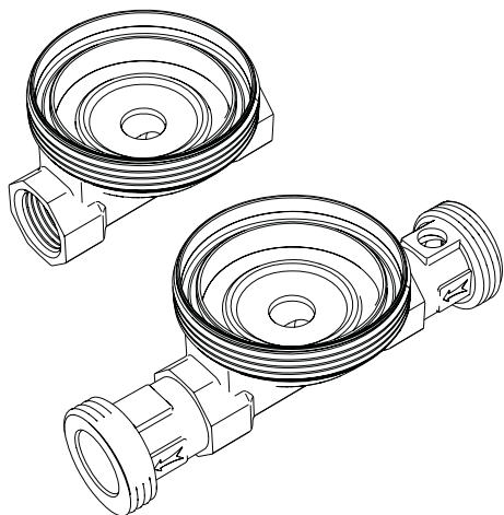
Рис. 13 Корпус насоса в стандартном исполнении и в исполнении "Х"
