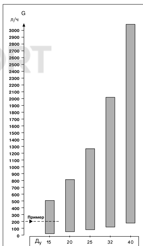
Рис. 5. Диаграмма для выбора диаметра клапанов серии ASV
