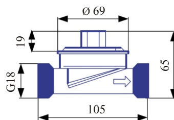
Рис.1 EAS с внешней резьбой
