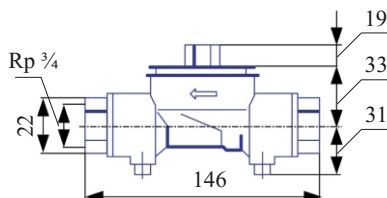
Рис.3 EAS с шаровыми кранами
