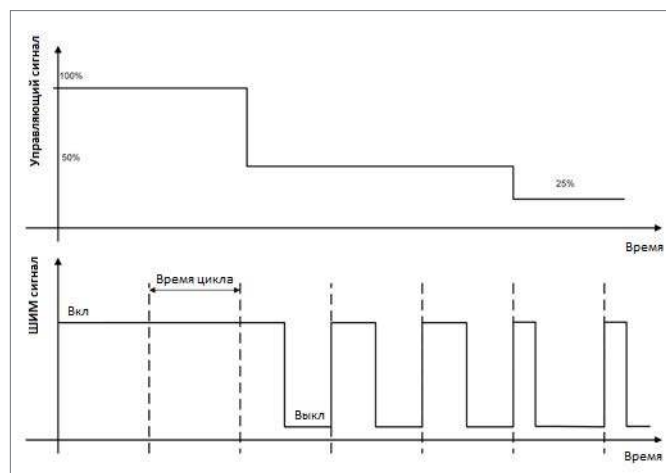
Abb. 4-3 Регулирующий сигнал и соответствующий сигнал ШИМ
