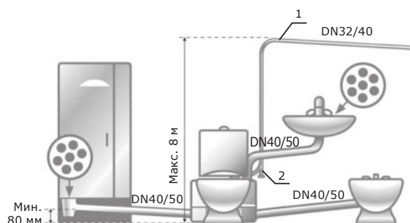
Рис. 30 Рекомендуемая схема монтажа напорного трубопровода
