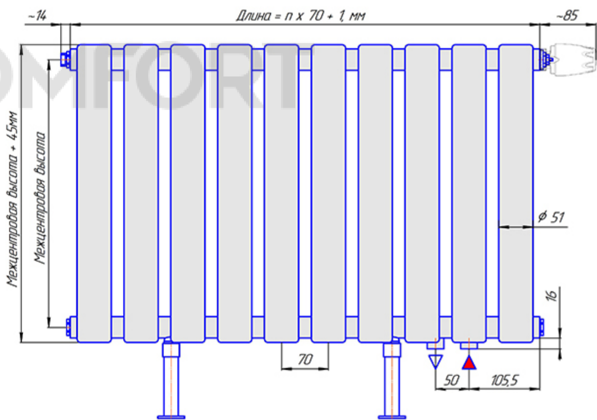
Присоединительная резьба - G 1/2" внутр.
