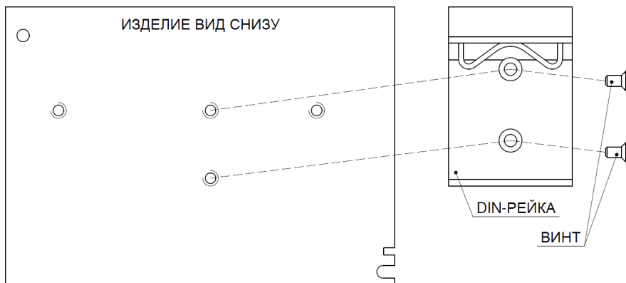
Рисунок 2 – крепление DIN-рейки.
