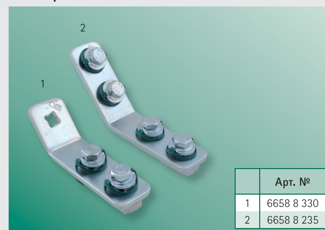
BIS RapidStrut® Уголки 135°
