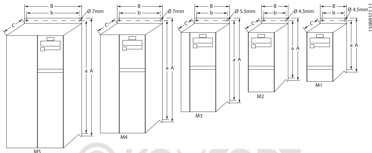
Рисунок 1.1 Габаритные размеры
