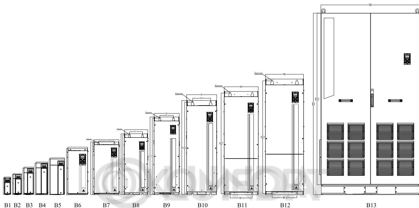
Рисунок 2.1-1 Типоразмеры преобразователей частоты
