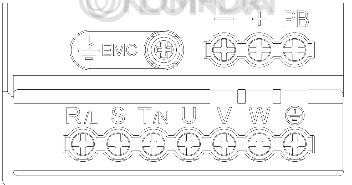
Рисунок 3.1-2 Расположение клемм
