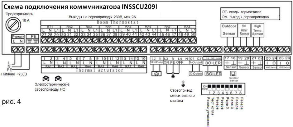
Схема электроподключений
