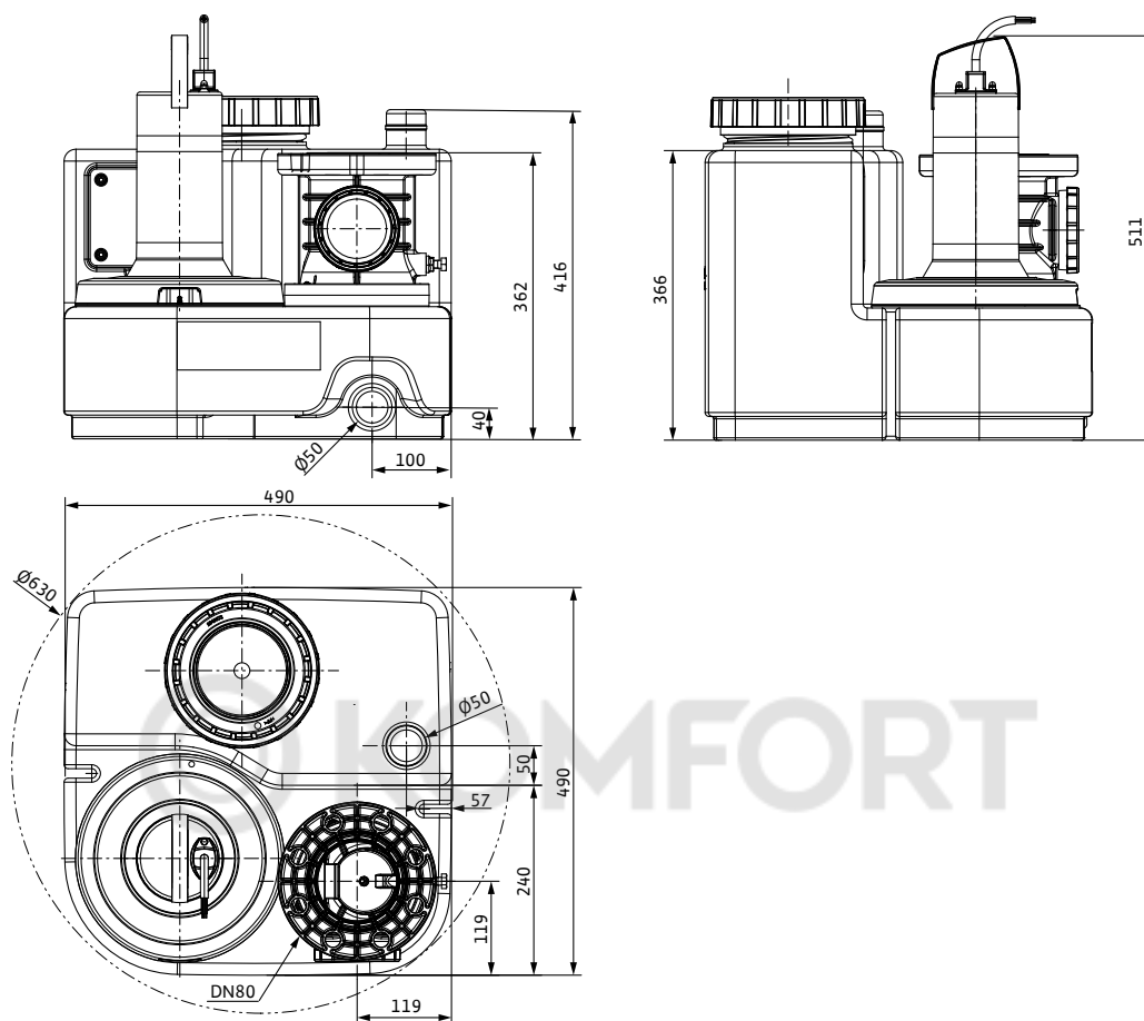
Габаритный чертеж DrainLift SANI-S
