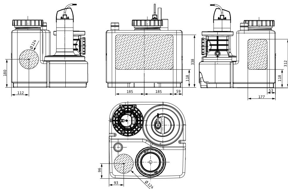
Габаритный чертеж DrainLift SANI-S. Место подсоединения приточного трубопровода
