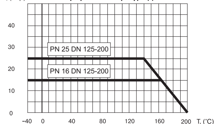
График «Температура-Давление»
