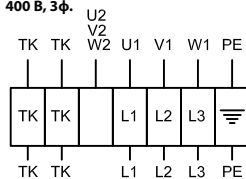
Схема 2 400 В, 3ф.
