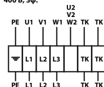
Схема 4 400 В, 3ф.
