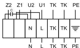
Схема 1 230В, 1ф
