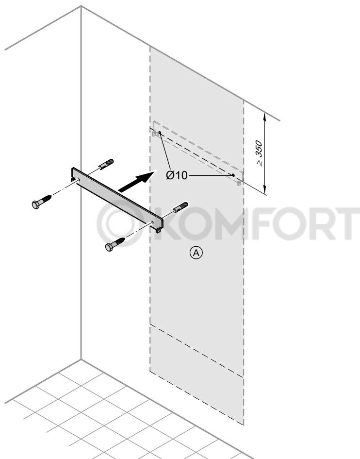
Ⓐ Монтажный шаблон
