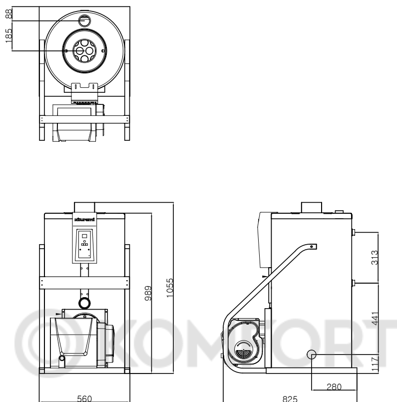
Рисунок 17. Габаритные и присоединительные размеры для котлов KSO-50
