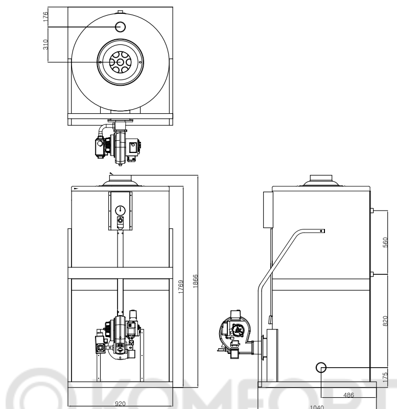
Рисунок 21. Габаритные и присоединительные размеры котлов KSO-200
