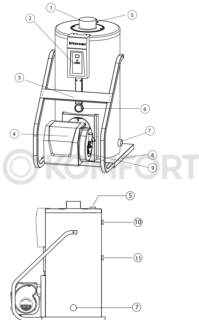
Рисунок 1. Устройство и назначение основных частей для котлов KSO- 50/70/100
