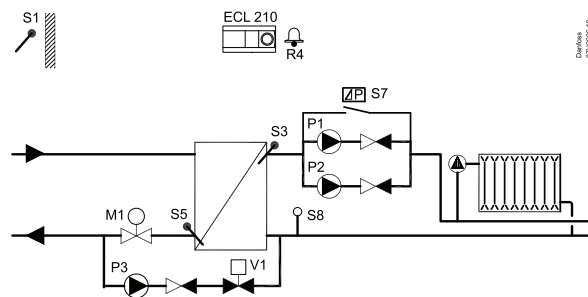
Стандартная схема A231.1:
