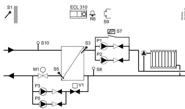
Стандартная схема A331.1:
