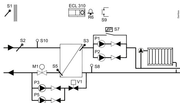
Стандартная схема A331.2:
