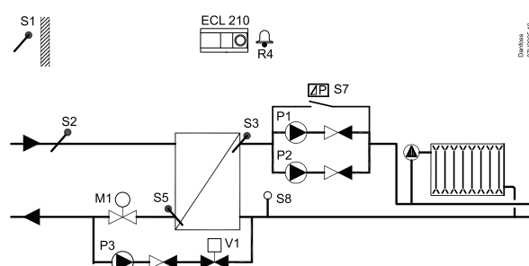
Стандартная схема A231.2:
