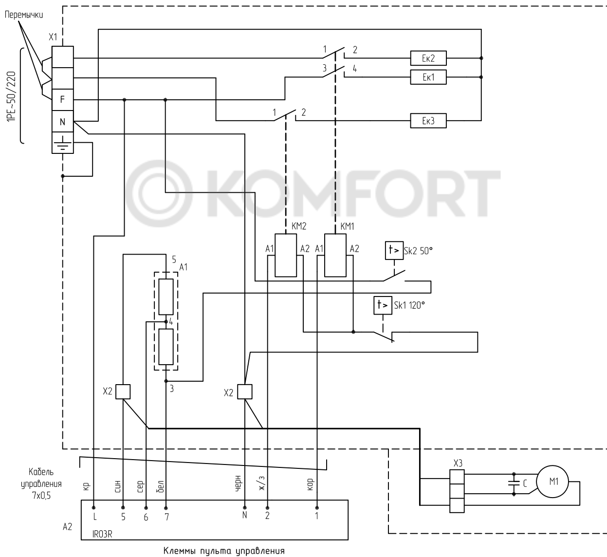
Рисунок 6. Электрическая схема занавеса КЭВ-6П2213Е
