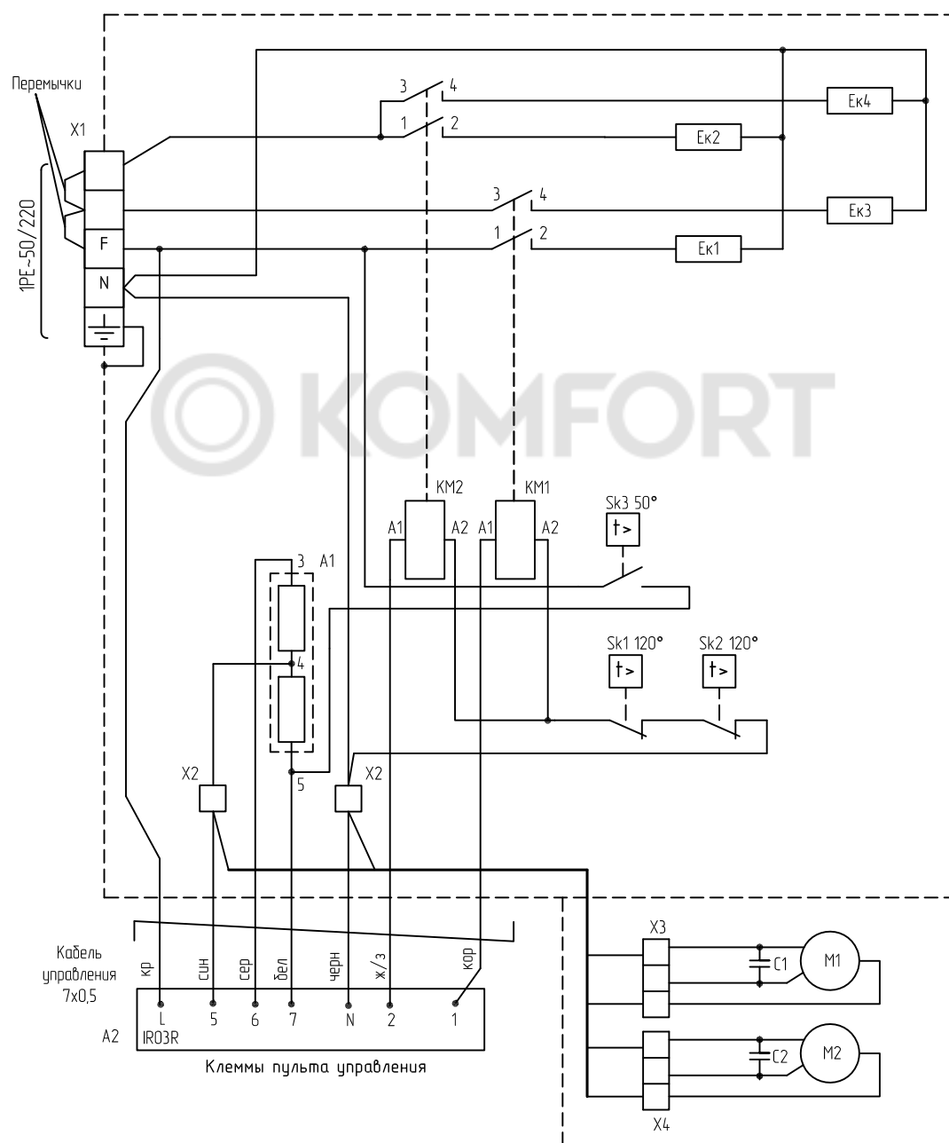
Рисунок 8. Электрическая схема занавесы КЭВ-6П2223Е
