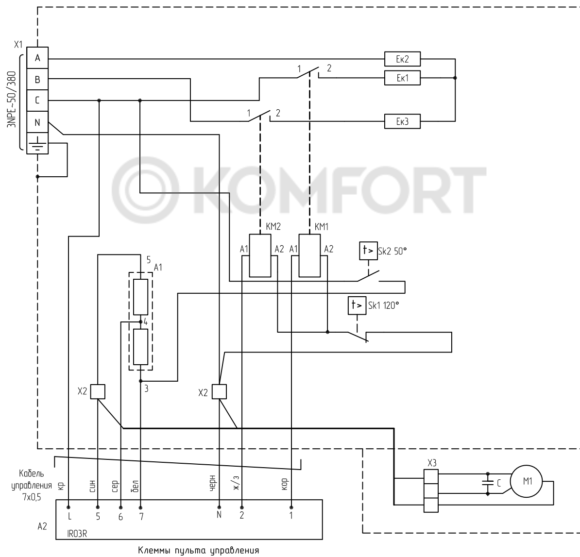
Рисунок 7. Электрическая схема занавесы КЭВ-6;9П2013Е
