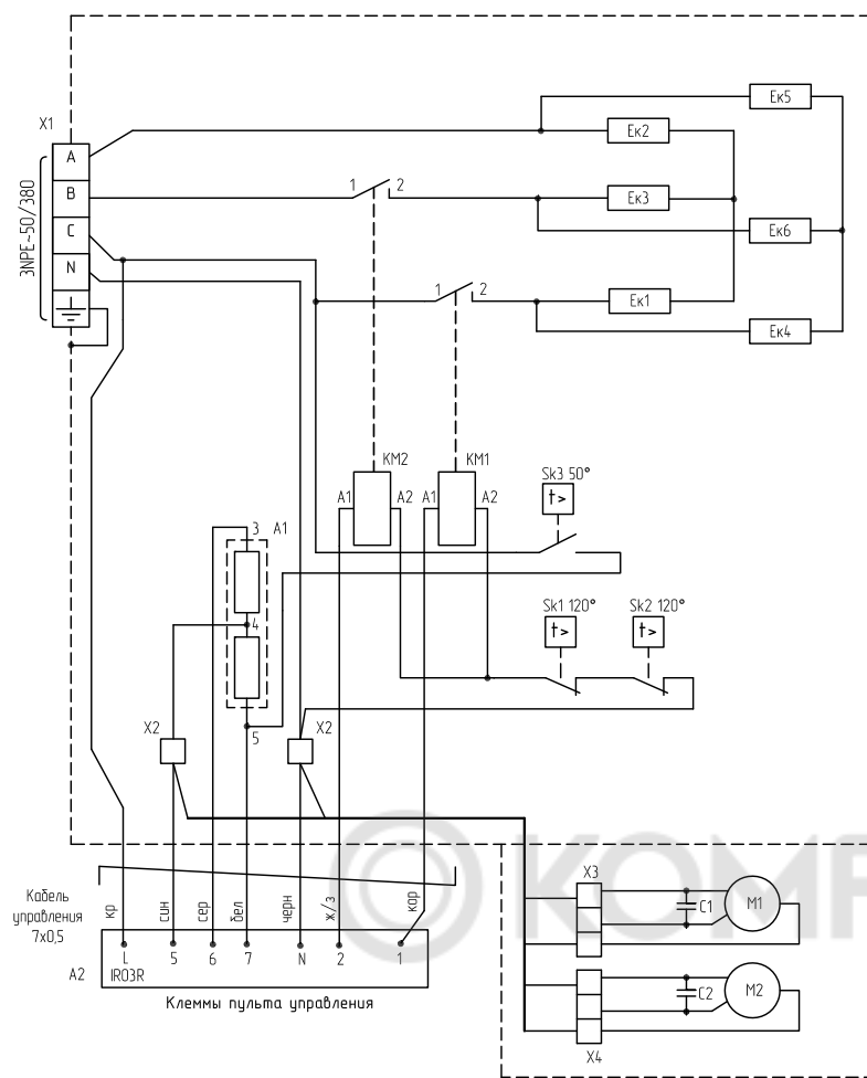
Рисунок 9. Электрическая схема завесы КЭВ-6;9П2023Е
