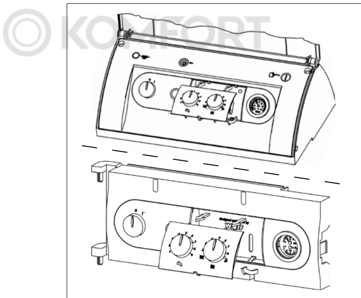
Рис. 4.8 Снятие передней панели
