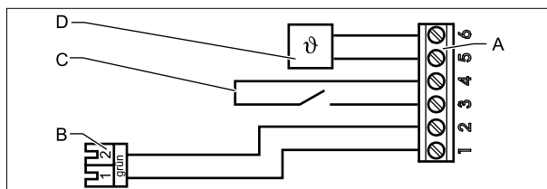
Рис. 4.6 Расположение блока клемм настенного цоколя
