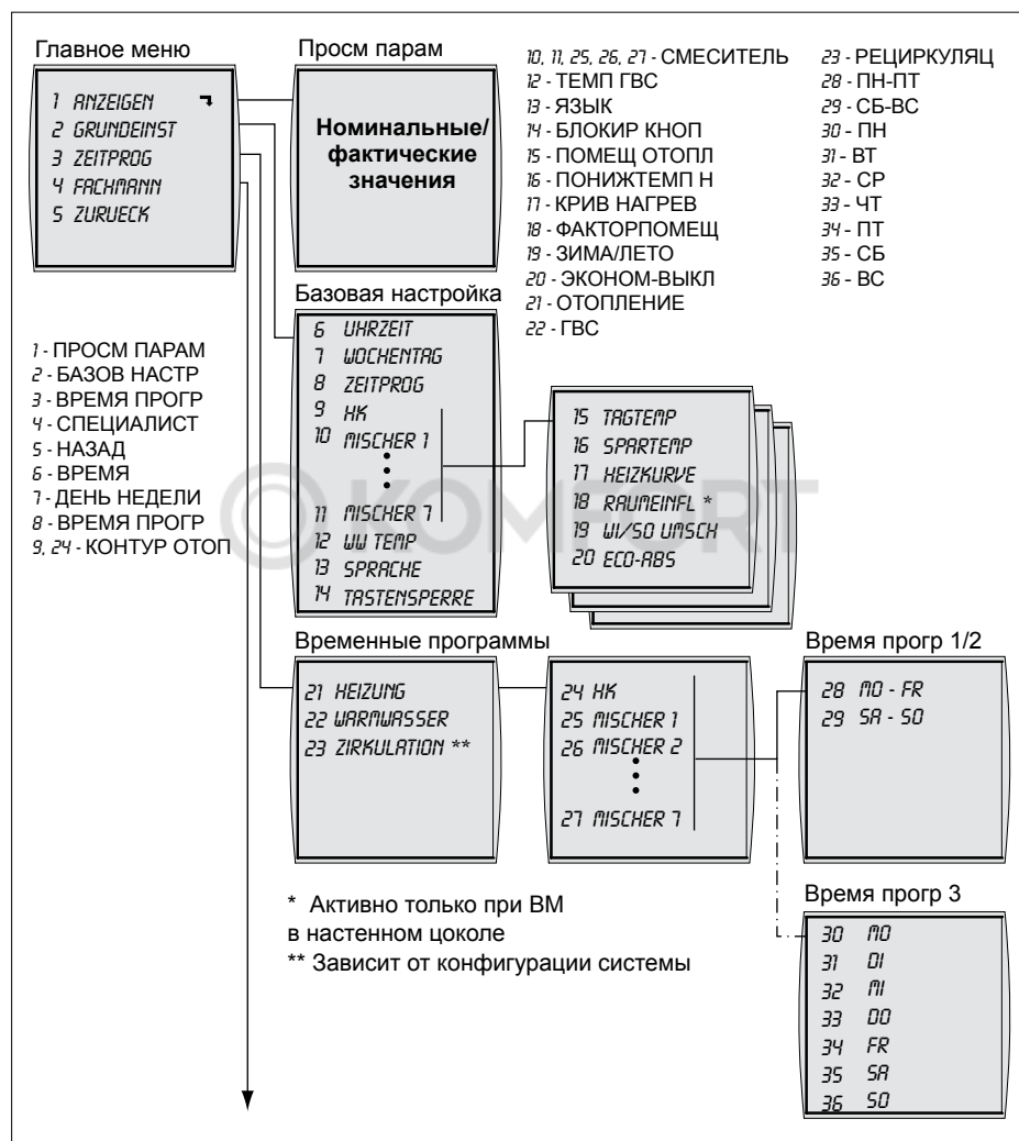
Рис. 5.2 Структура меню модуля управления ВМ
