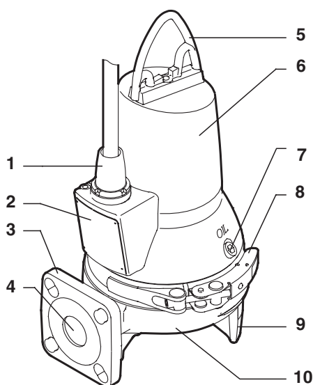
Рис. 1 Насос SEG
