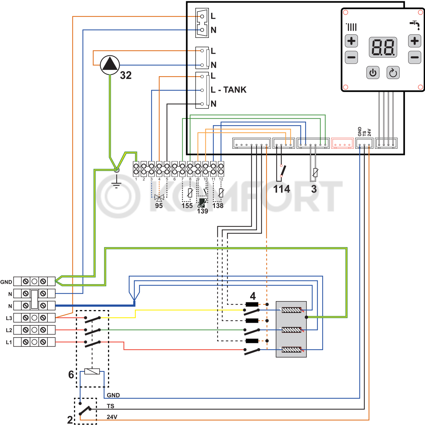
Рис. 17. Для моделей 6, 9 и 12 кВт
