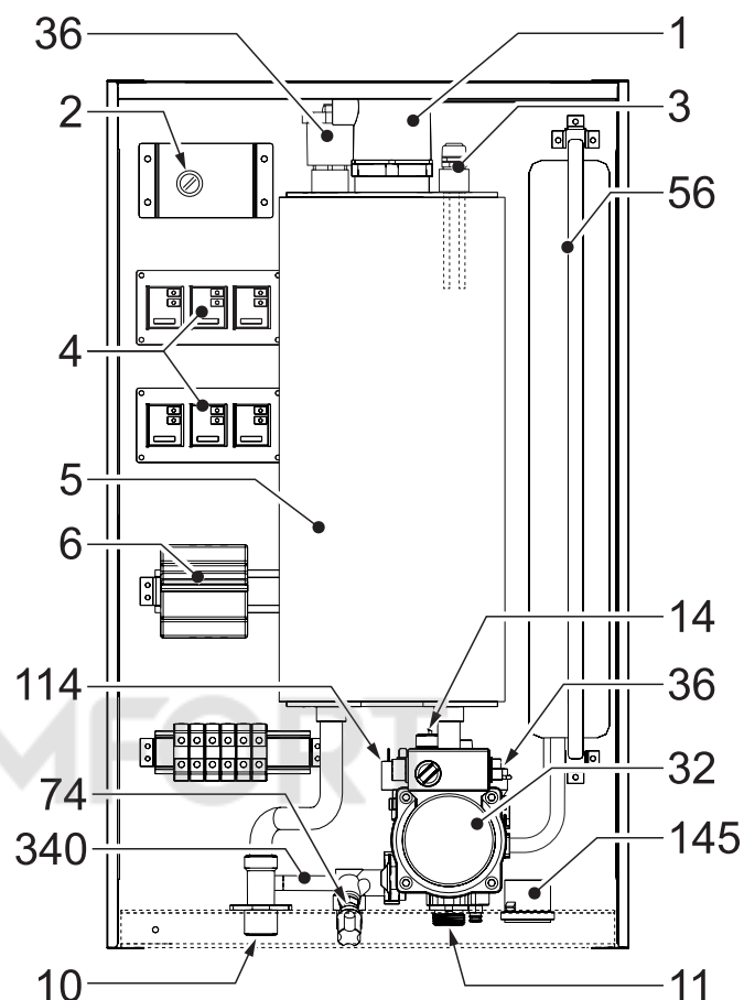
Рис. 15 TOR 15-24 кВт
