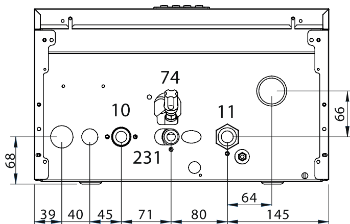
Рис. 12. Вид снизу
