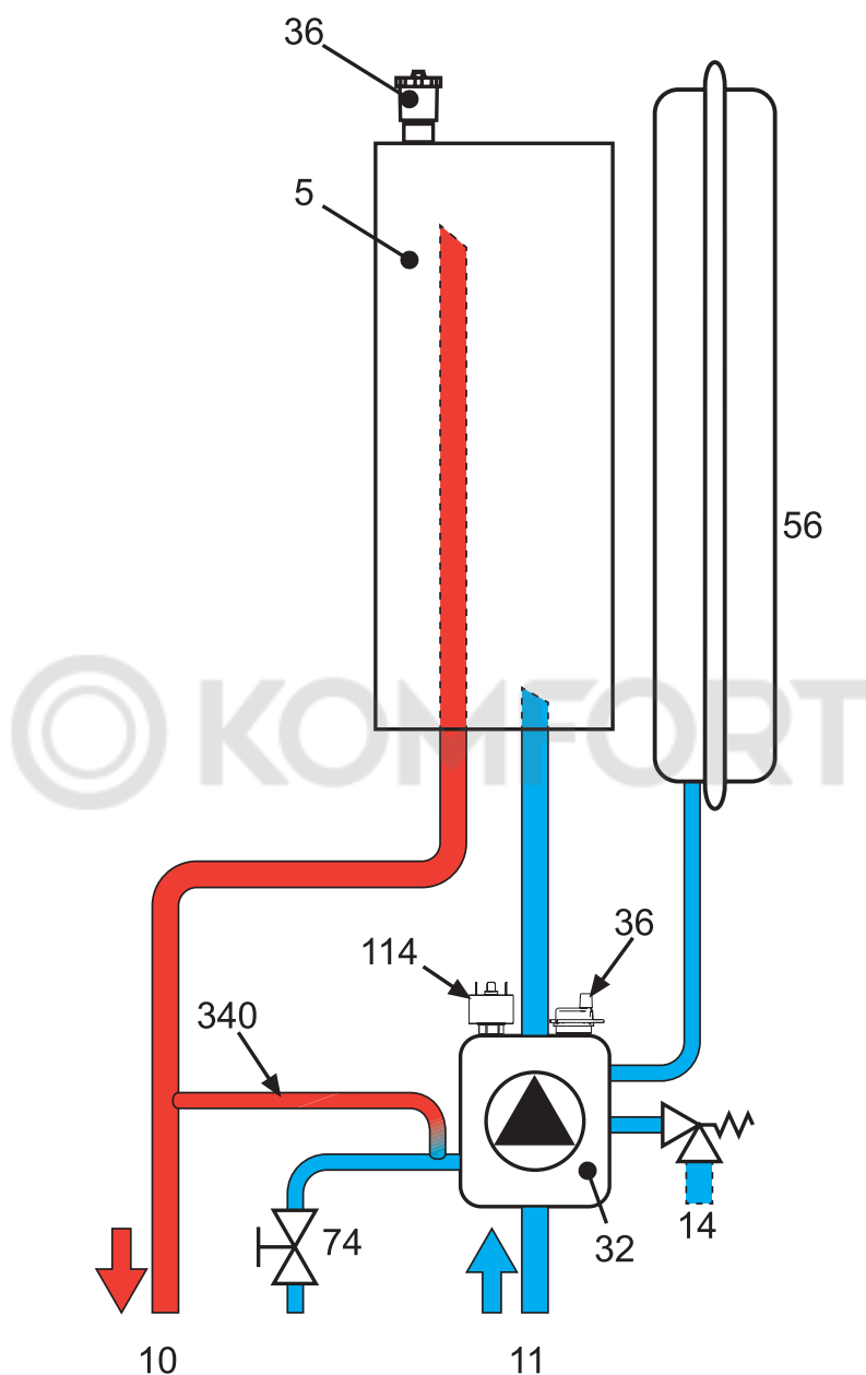
Рис. 16 Гидравлическая схема
