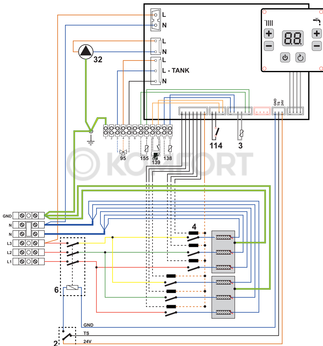
Рис. 18. Для моделей 15, 18, 21 и 24 кВт
