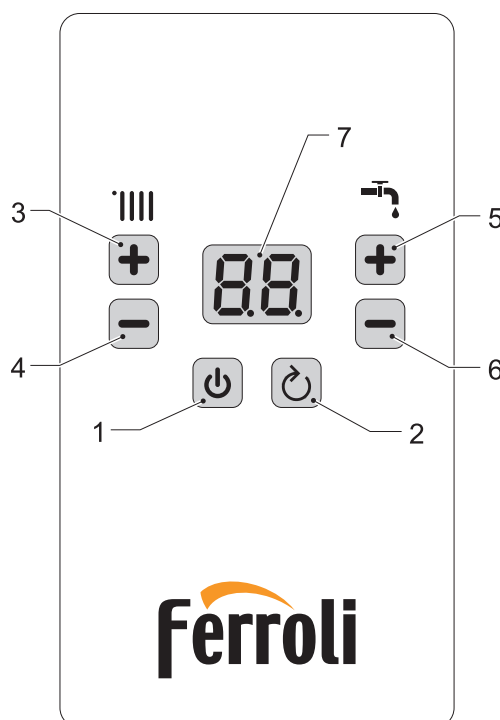
Рис. 1. Панель управления
