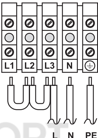
Рис. 20. Однофазная проводка
