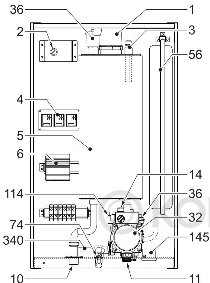
Рис. 14 TOR 6-12 кВт
