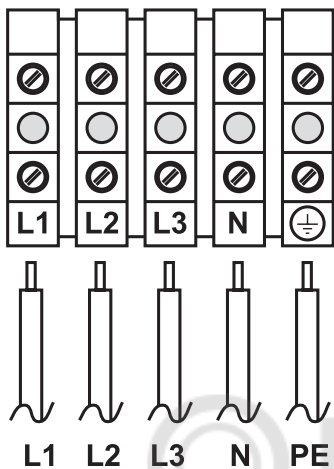
Рис. 19. Трехфазная проводка
