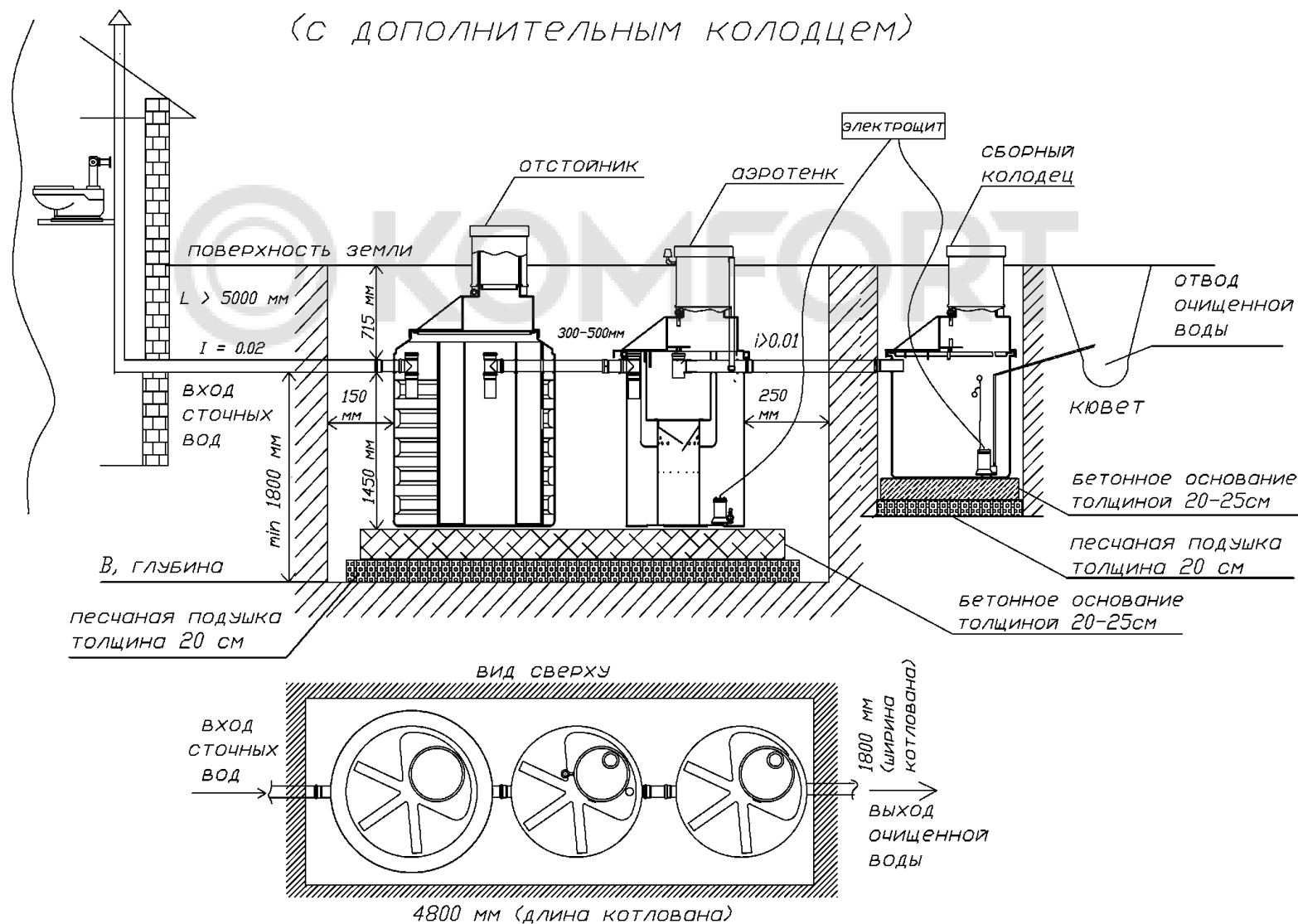
6.2. Монтажная схема ЛОС 5, 8 со сборным колодцем (плывун)
