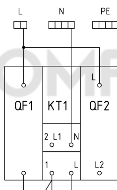
Рис. 9.2 Монтажная схема щита управления установки ЛОС 8.
