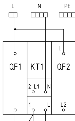
Рис. 9.1 Монтажная схема щита управления установки ЛОС 5.
