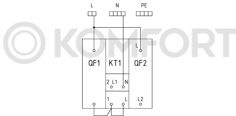
Рис. 9.2 Монтажная схема щита управления установки ЛОС 8.
