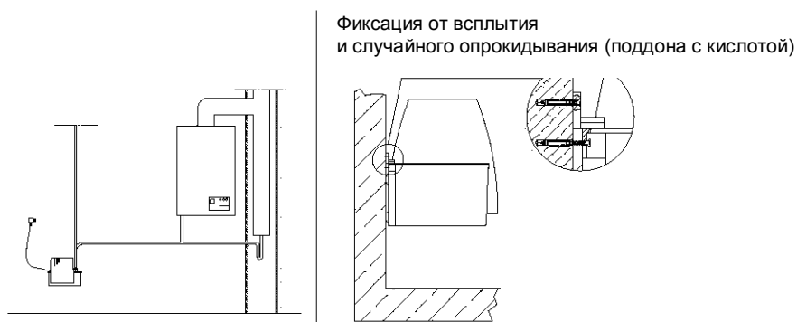
Рис. 4 Настенный монтаж с применением прихватов-угольников
