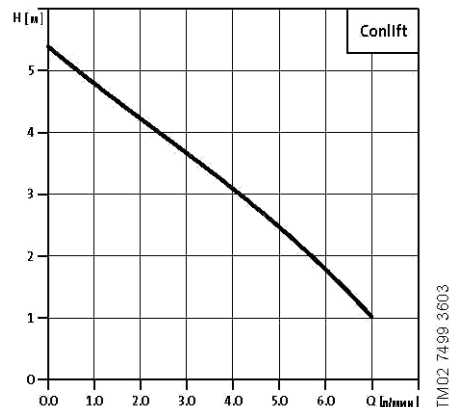
Рис. 9 График характеристики
