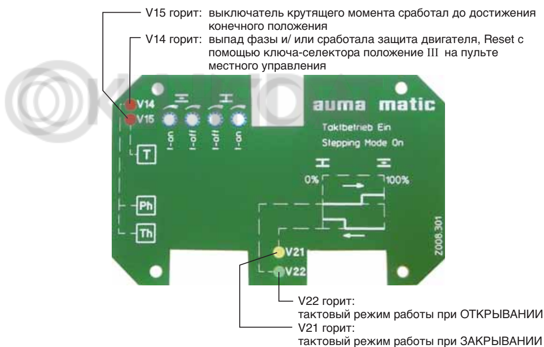
рис. U-1: Защитная плата тактового датчика A1.6
