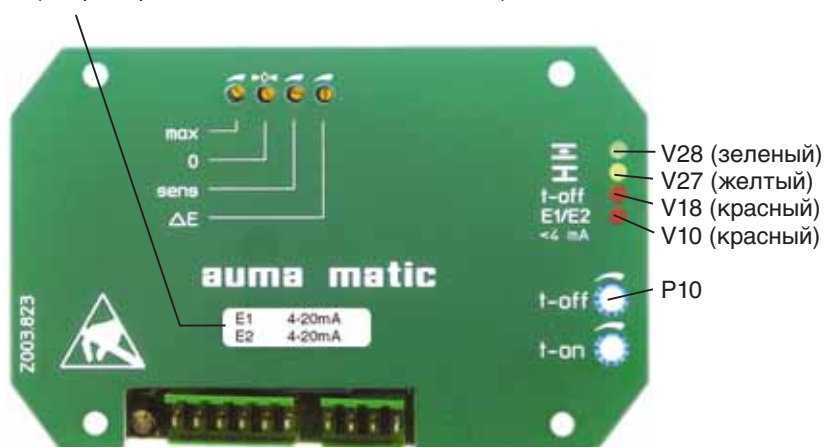
рис S2: Плата регулятора положения A7
