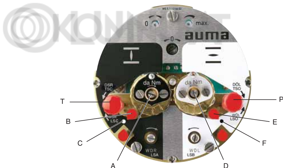
рис. К-1: Блок выключателей
