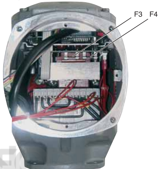
рис. V2: Предохранители на плате блока питания
