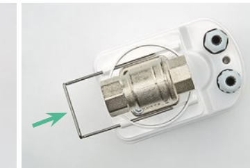
Фото 6. Крепление электропривода к шаровому крану с помощью металлической скобы
