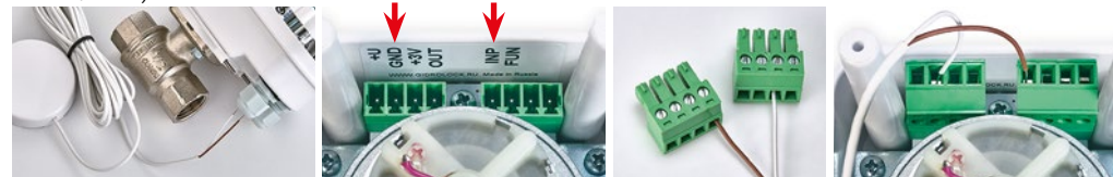
Фото 12. Завести провод датчика в кабельный ввод
