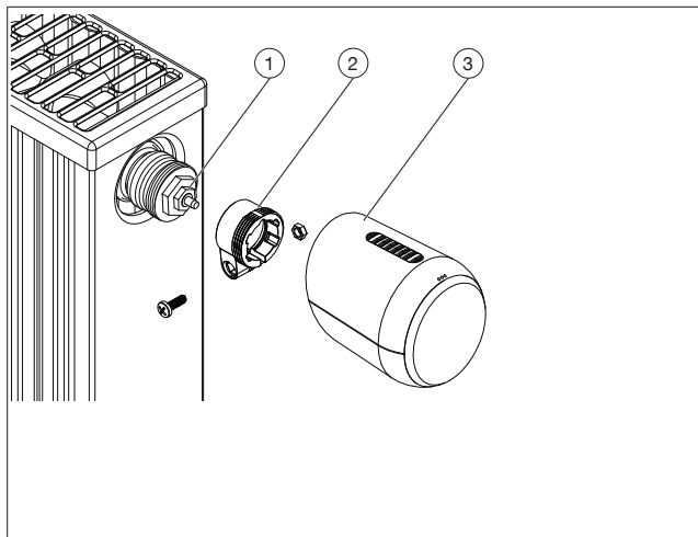
Рис. 4: монтаж „mote 200“
