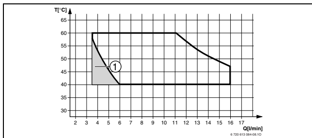
Рис. 13 Диаграмма температуры подаваемой холодной воды от +15\text{ °C} (ZWC 35)
