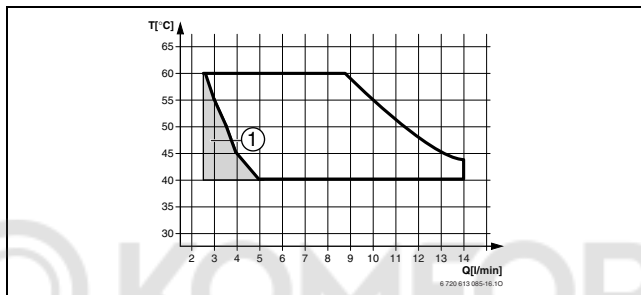
Рис. 12 Диаграмма температуры подаваемой холодной воды от +15\text{ °C} (ZWC 28)
