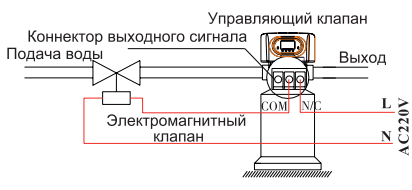
Рис. 3-2 Цепь управления электромагнитным клапаном на входе
