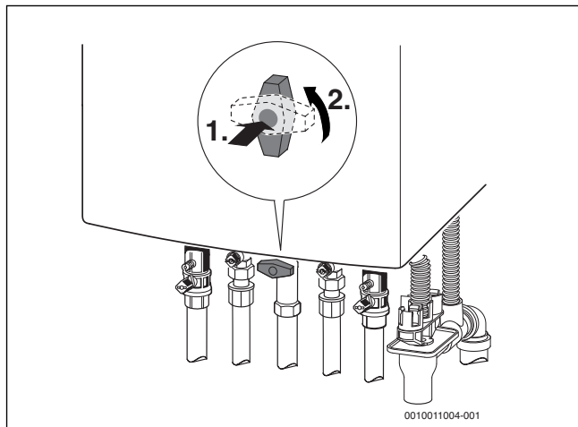
Рис. 2 Открытие газового крана
