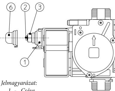
SIT 845 gázszelep
