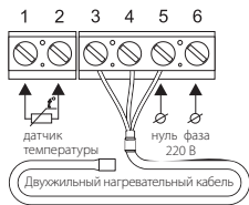
Схема подключения к 2-х проводной электрической сети
