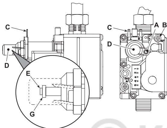
Рис. 15. Газовый клапан
