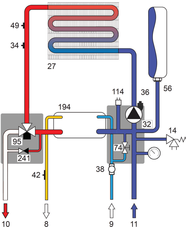
Рис. 19. Контур ГВС
