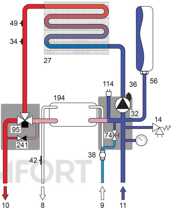
Рис. 18. Отопительный контур
