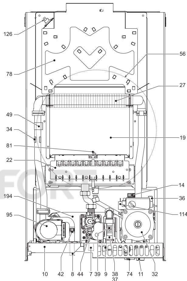
Рис. 17а. Конструкция Fortuna C32
