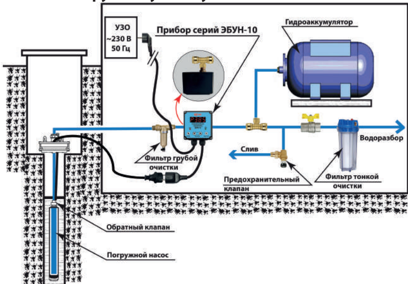
Пример 2. Подключение приборов серии ЭБУН-10 к погружному насосу.
