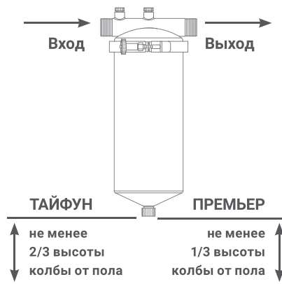
Рис. 1. Подключение фильтра.
